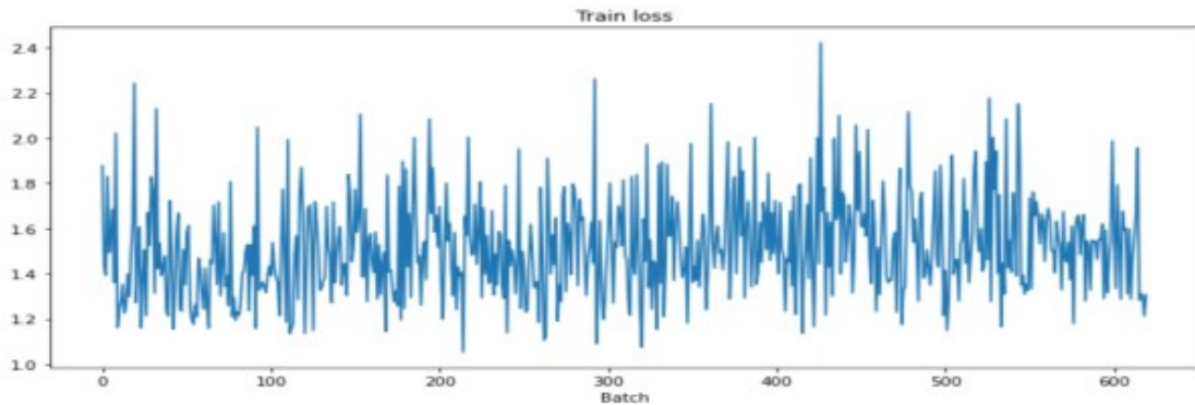
Рисунок 3 - График изменения ошибки во время обучения нейронной сети
