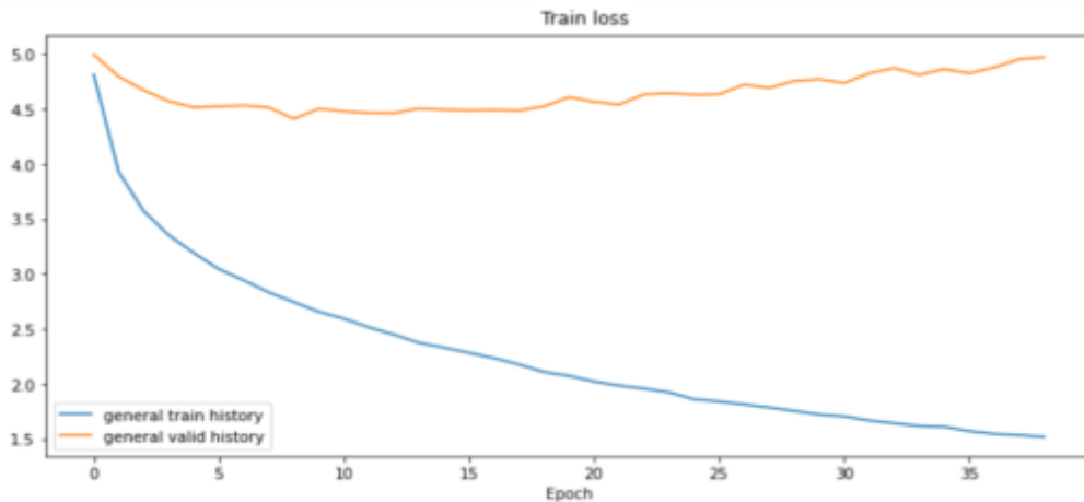
Рисунок 4 - График изменения ошибки обучения от количества эпох
