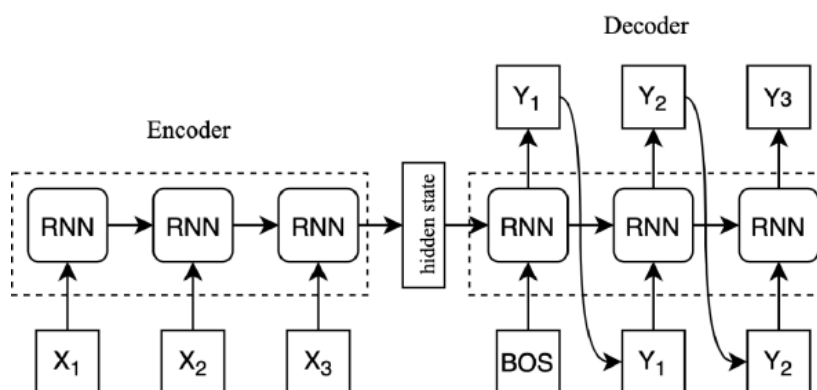
Рисунок 1 – Sequence-to-sequence модель для машинного перевода
